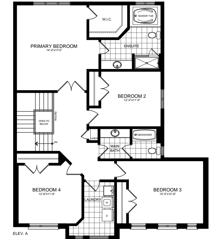
ELEV. A
