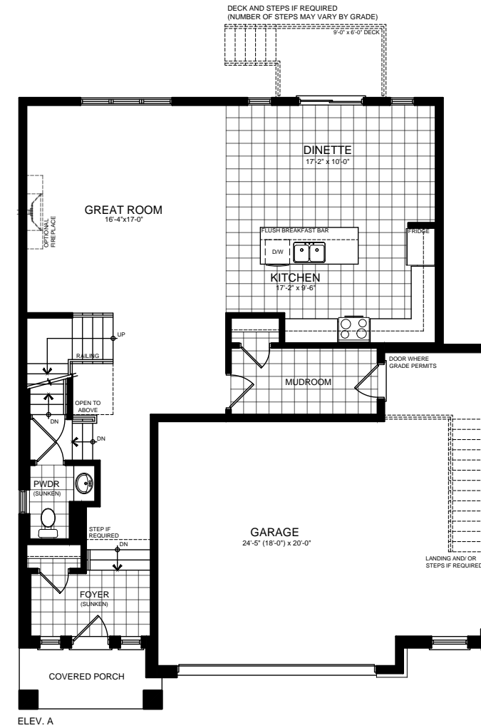
ELEV. A
